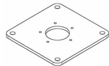
Mounting plate „M4“ (1)
